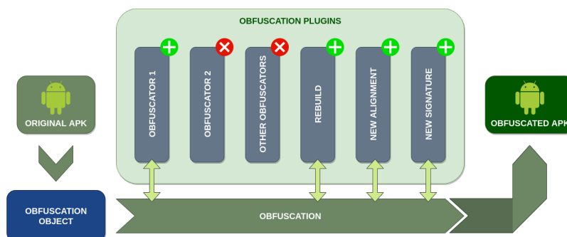
شکل ۷-۱: شمای کلی برنامه obfuscapk جهت مبهم سازی برنامه‌های آندروید
